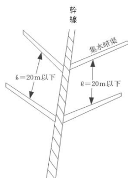
図 2 集水暗渠の施工間隔
