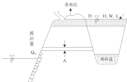
図3 遊水池の考え方
