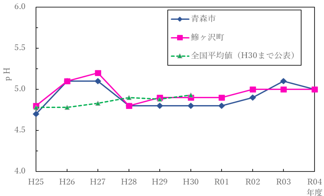
図2 酸性雨経年変化
