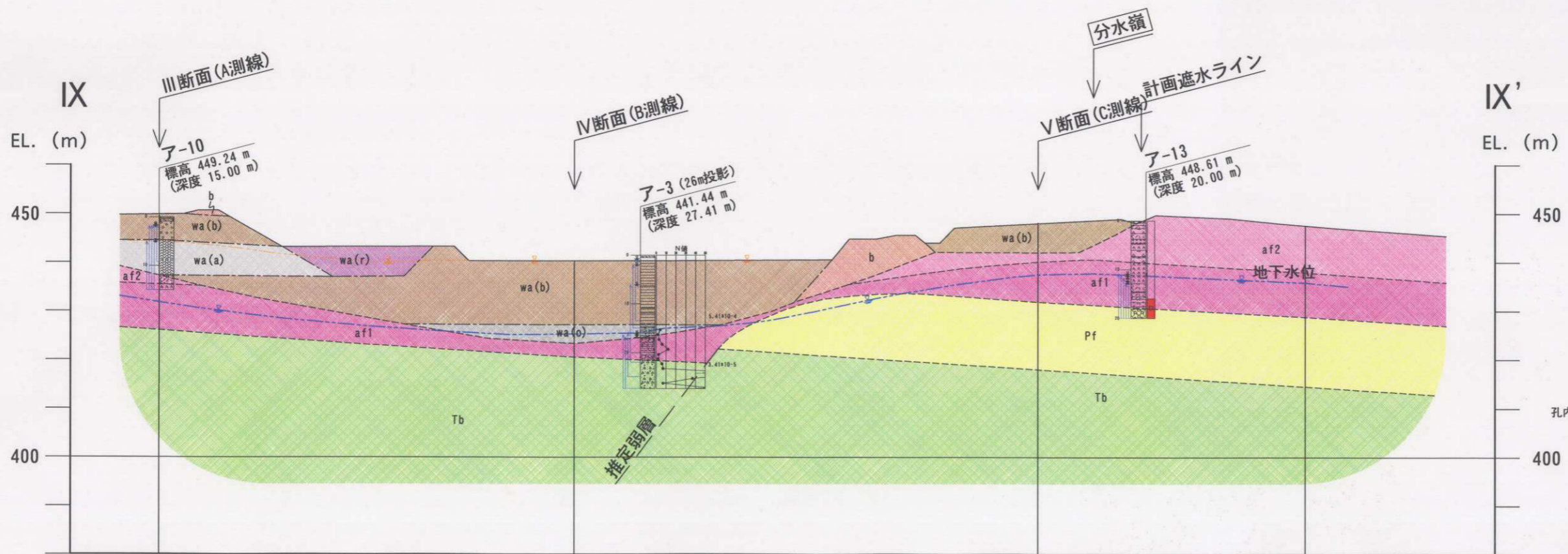
図-3 I 断面・IX断面 地質断面図
