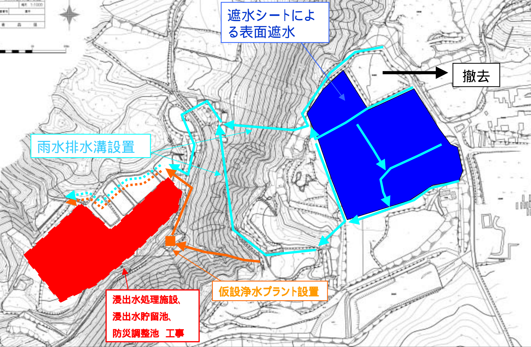
図3-3 仮設浄水プラント配置図
