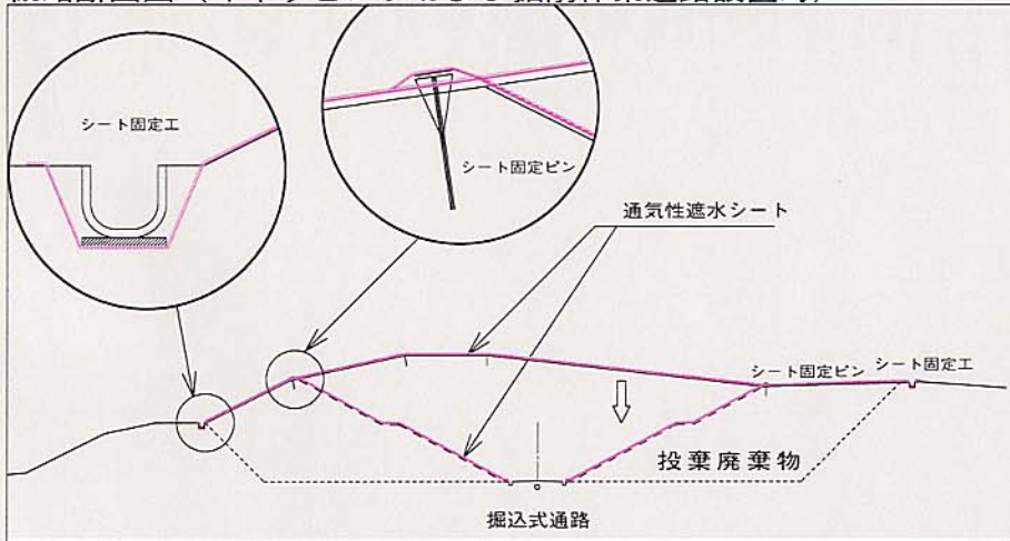
概略断面図（廃棄物撤去完了時）
