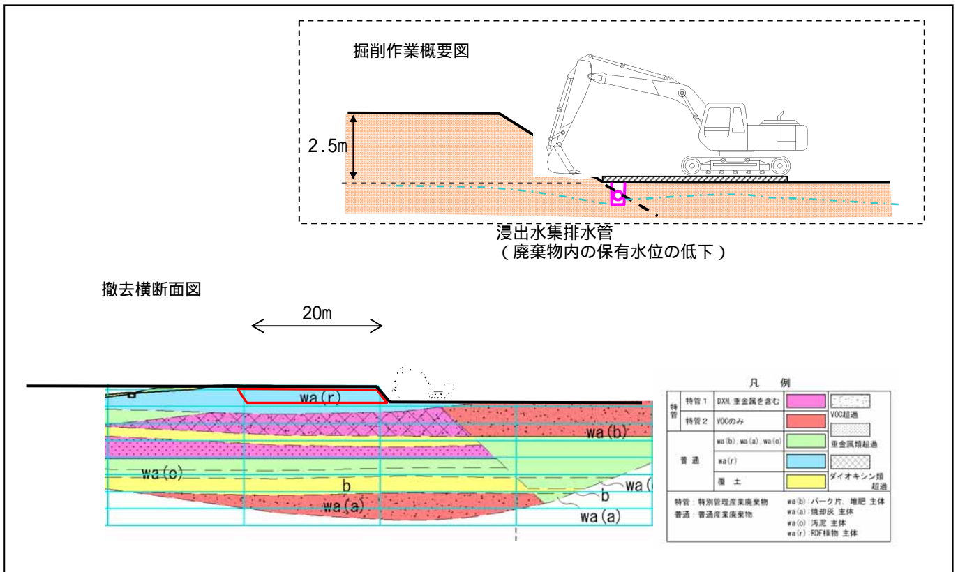
図 3-1 掘削標準図
