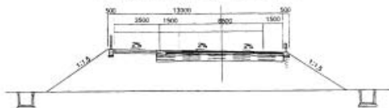
■標準断面図(一般部)■
