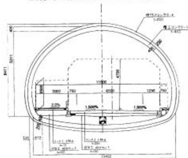
■標準断面図(トンネル部)■
