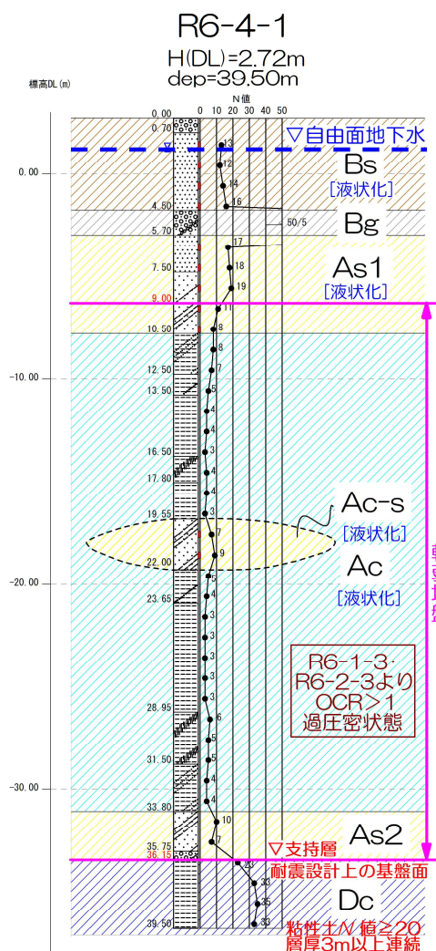
推定地層断面図
