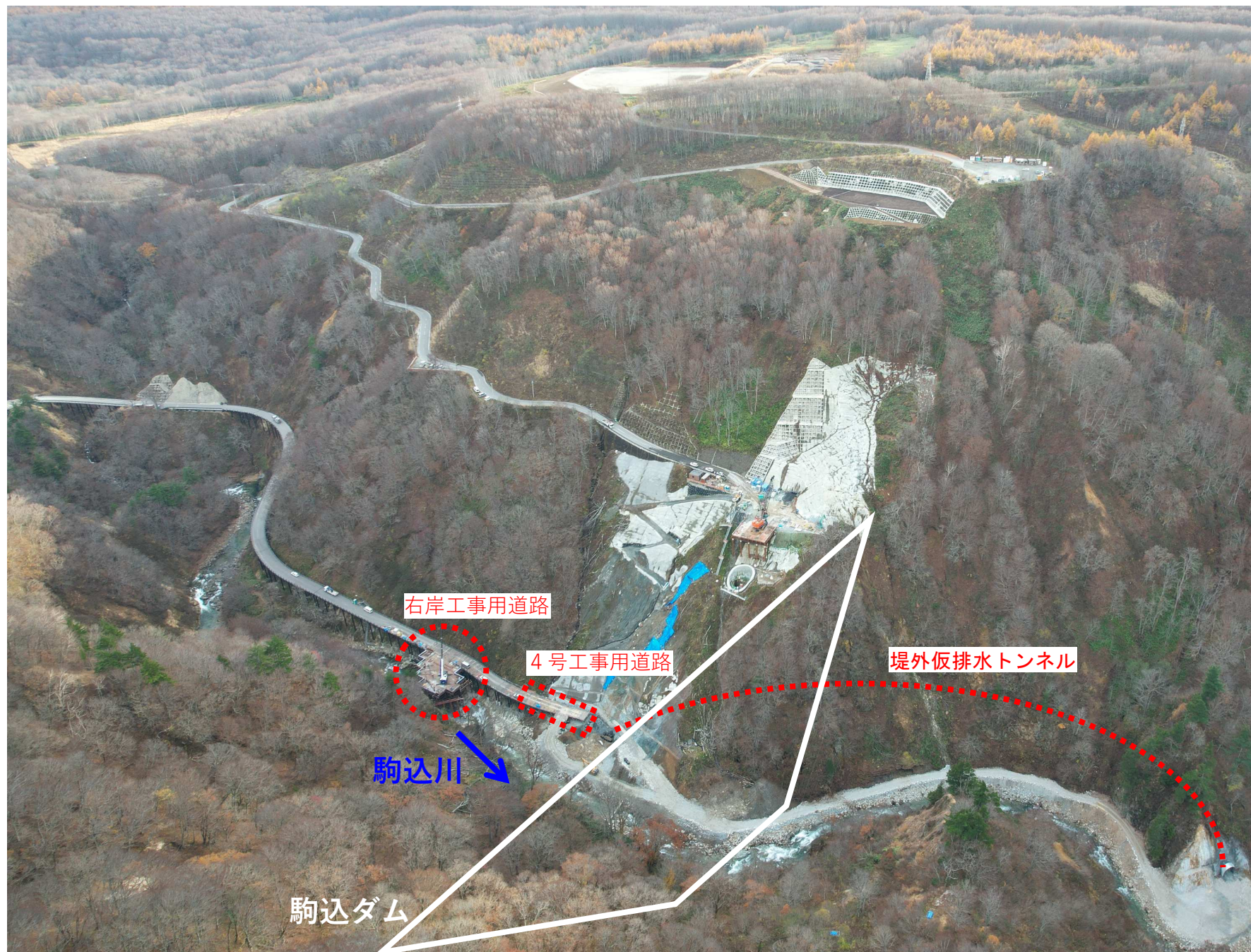
(1)ダム建設予定地全景 (R4年11月撮影)
