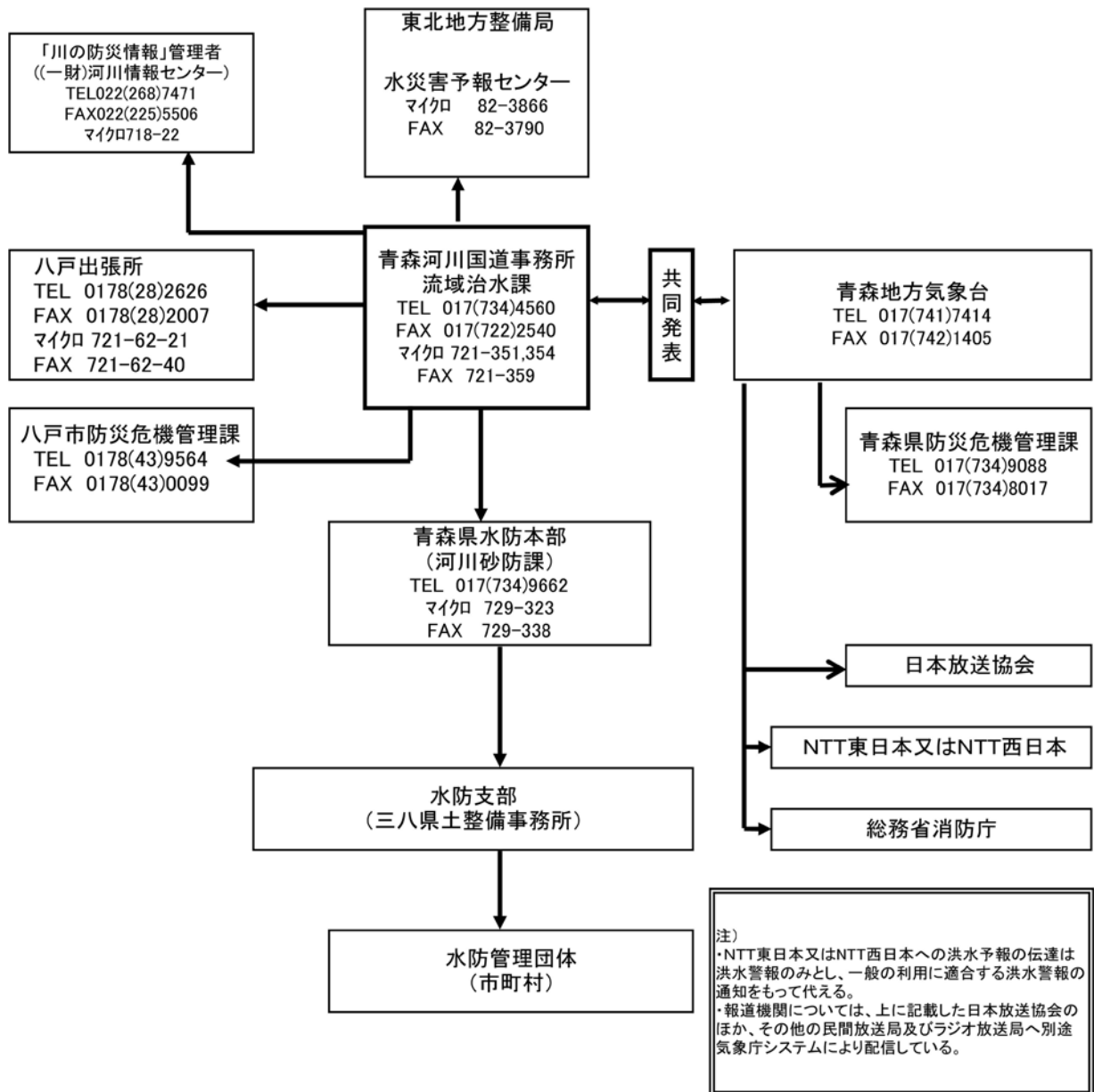
② 馬淵川下流洪水予報伝達系統図
