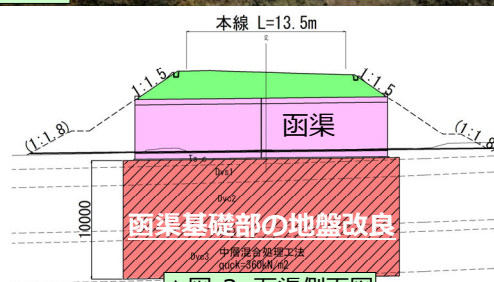
▲図-3 函渠側面図
