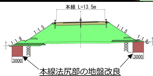
▲図-2 本線標準横断面図
