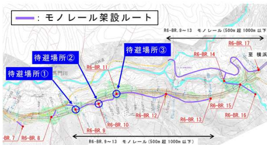
牽引車待避場所位置図
