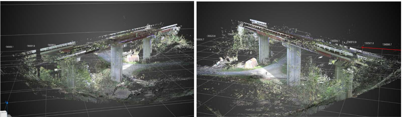
地上レーザースキャナによる点群データ
