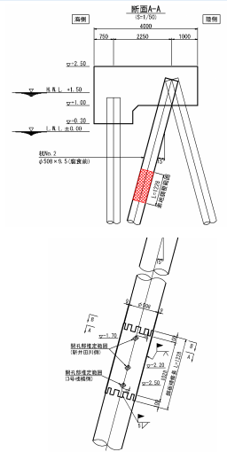
鋼板溶接補修の例
