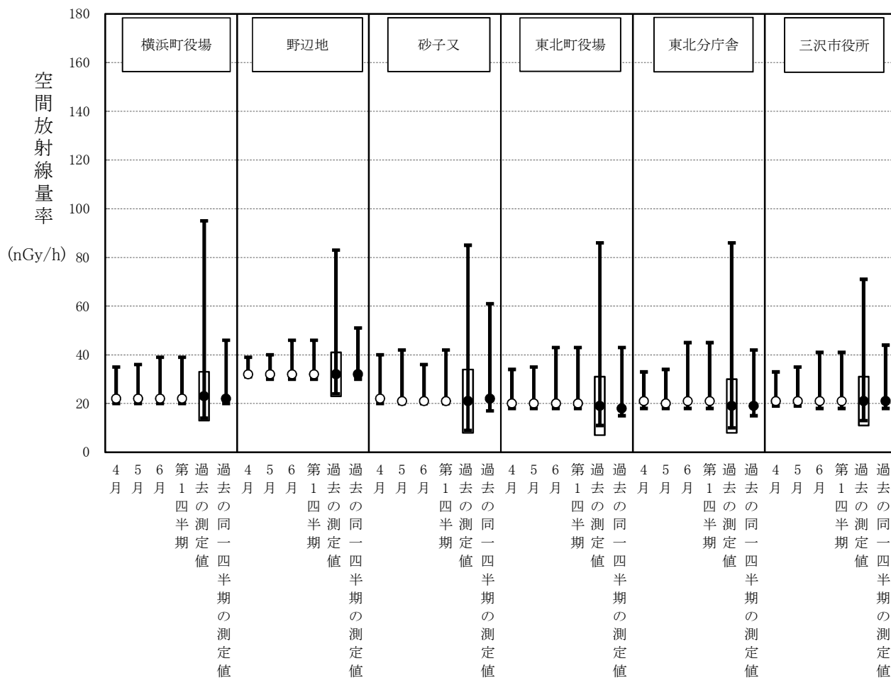
図2-2 モニタリングポストによる空間放射線量率(NaI)測定結果
