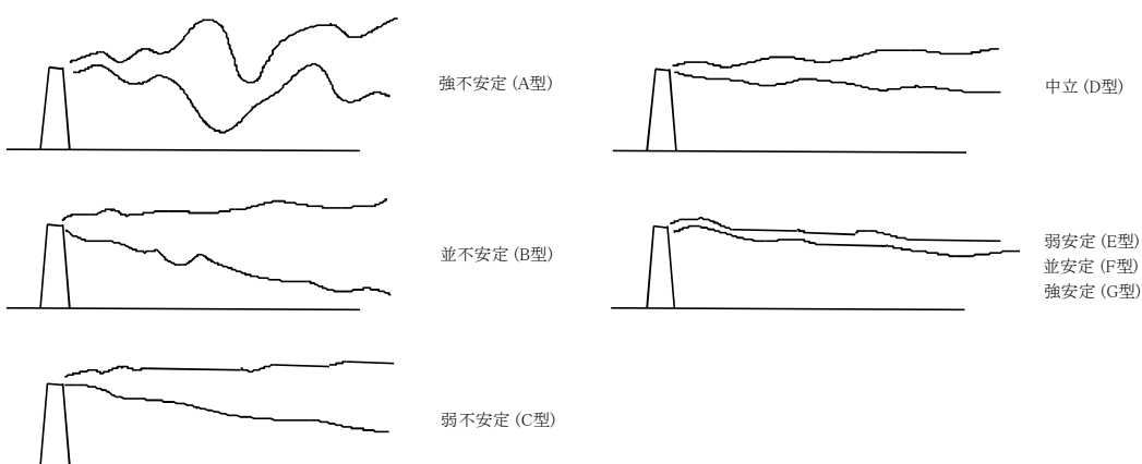
大気安定度と煙の型との模式
