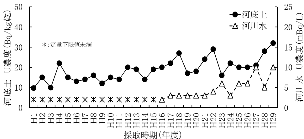
図 1 河底土及び河川水(二又川下流)ウラン濃度の推移
