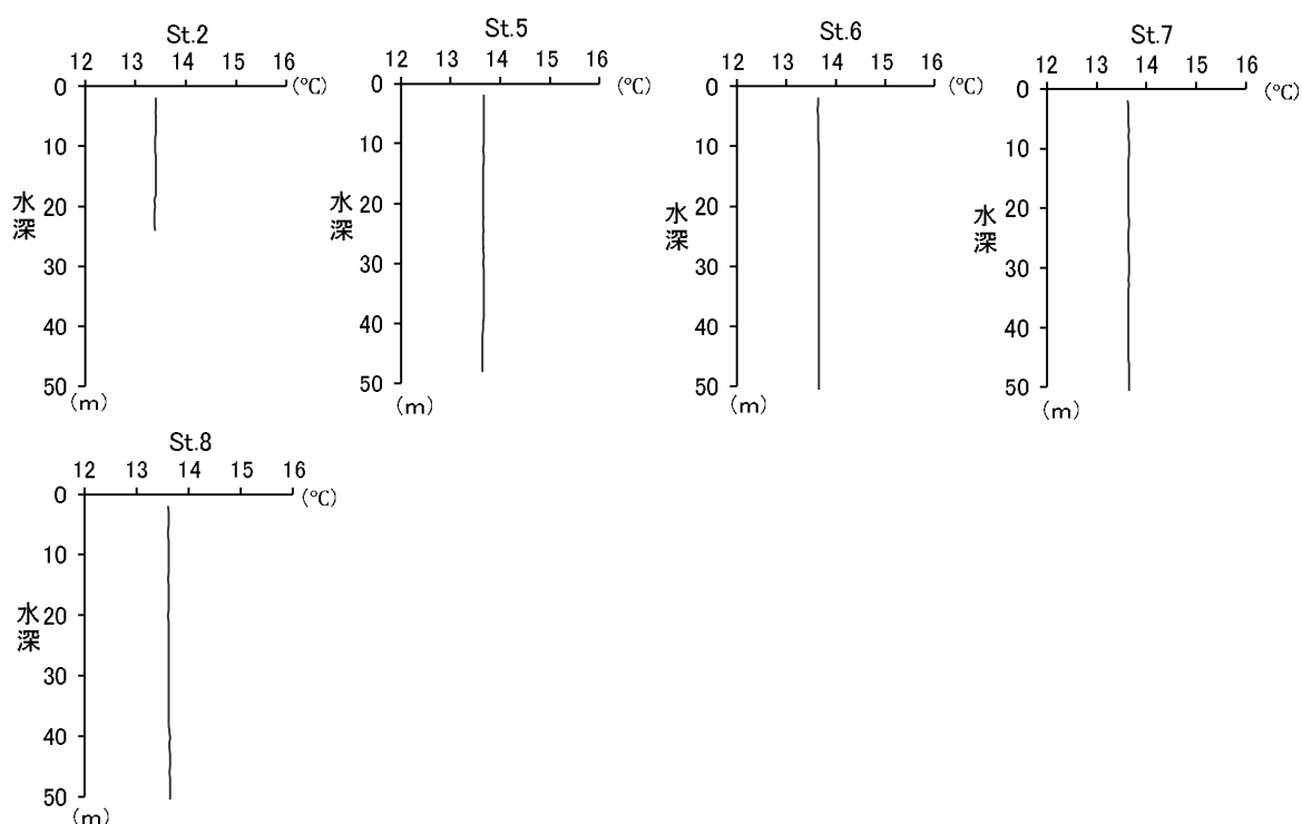
図-2.3 (3.2) 水温鉛直分布図 (全体)
