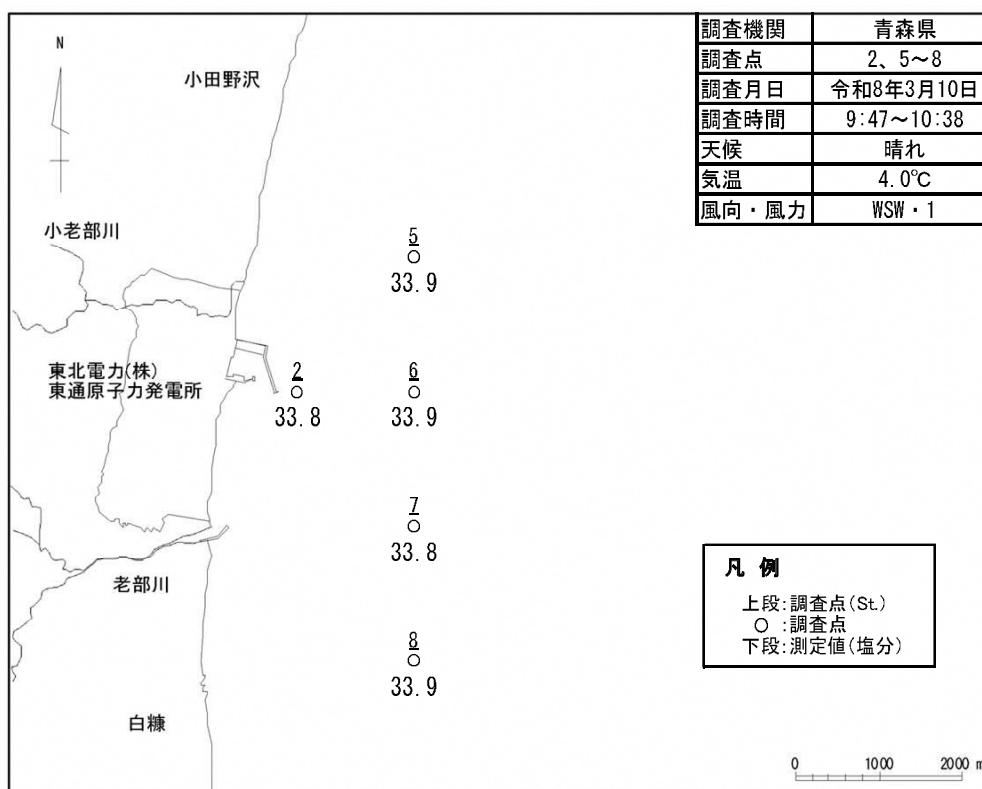
図-2.4 (2) 塩分水平分布図 (表層)
