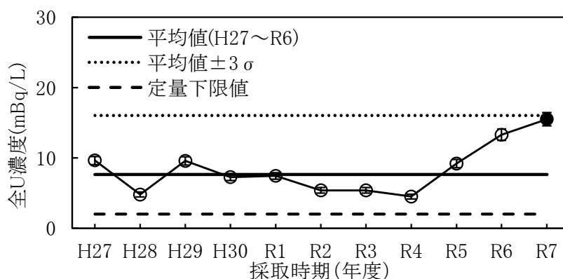
図 1 河川水(二又川)全 U 濃度の推移
