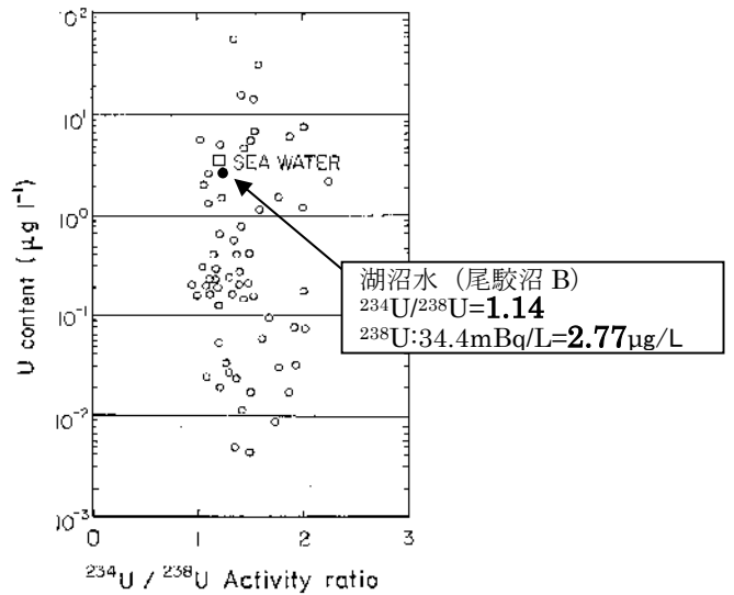
図 3 地表水の ^{234}\text{U}/^{238}\text{U} 放射能比と 全ウラン濃度 [1]
