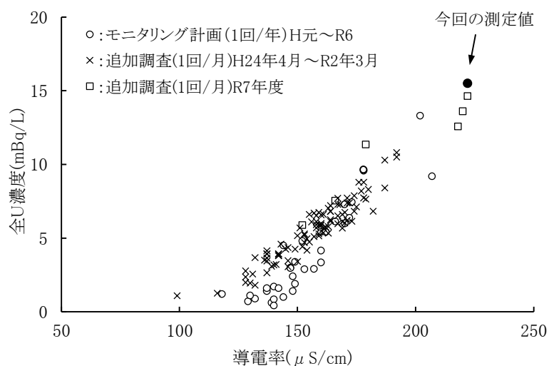
図4 導電率と河川水(二又川)中全 U 濃度との関係
