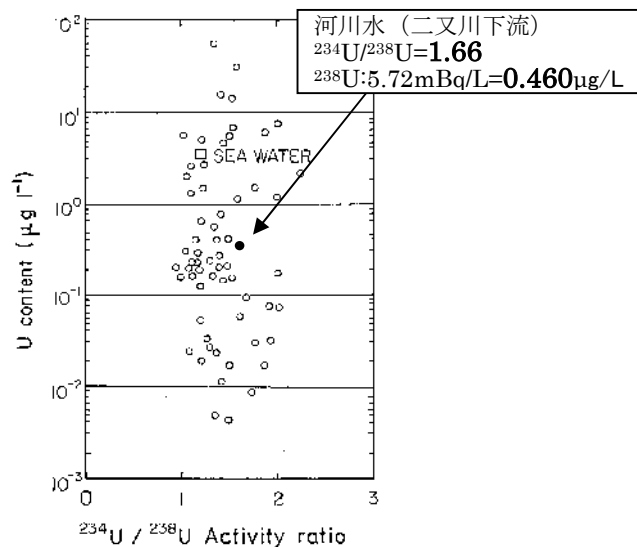
図3 地表水の ^{234}\text{U}/^{238}\text{U} 放射能比と全ウラン濃度 [1]
