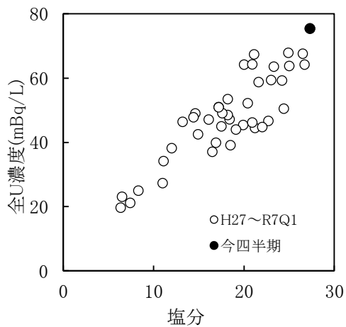
図 4 塩分と湖沼水(尾駁沼 B)中 全 U 濃度の関係
