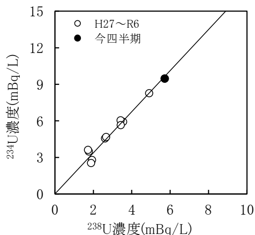
図2 河川水(二又川)中 ^{234}\text{U} と ^{238}\text{U} 放射能濃度の関係
