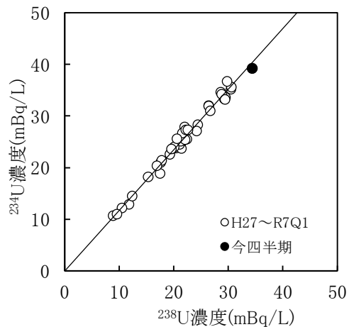
図 2 湖沼水(尾駁沼 B)中 ^{234}\text{U} 濃度と ^{238}\text{U} 濃度の関係
