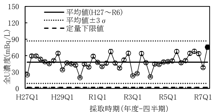
図 1 湖沼水(尾駁沼 B)全 U 濃度の推移
