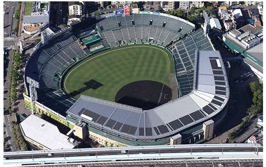
参考事例 阪神甲子園球場 (銀傘への太陽光発電敷設・年間19.3万kWhを発電) 【写真提供：阪神電気鉄道株式会社】
