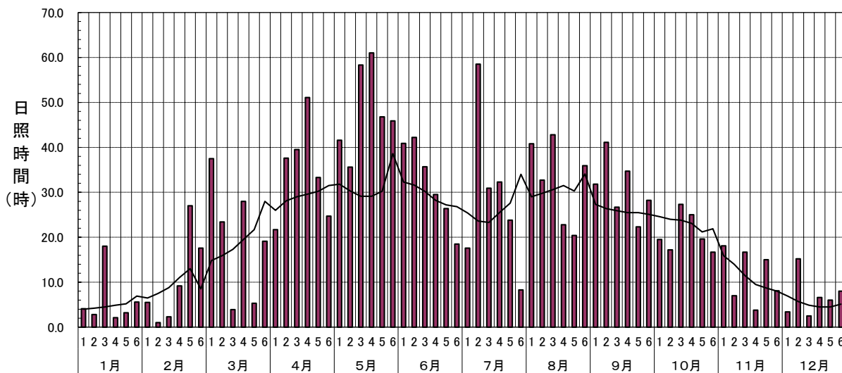
半旬別気象図 日照時間(市浦:2019年)
