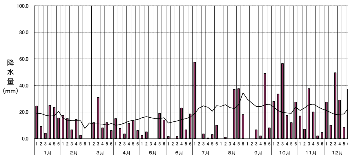
半旬別気象図 降水量(市浦:2019年)
