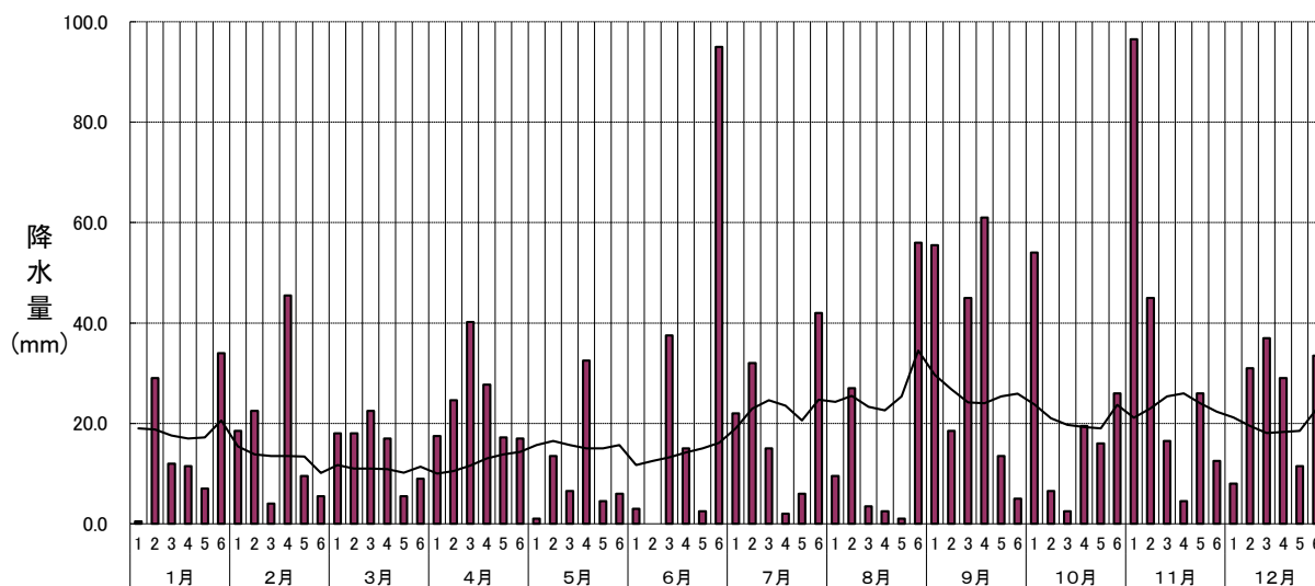
半旬別気象図 降水量(市浦:2020年)
