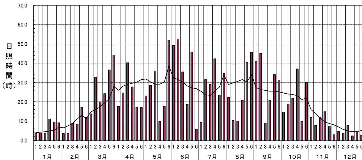
半旬別気象図 日照時間(市浦:2020年)
