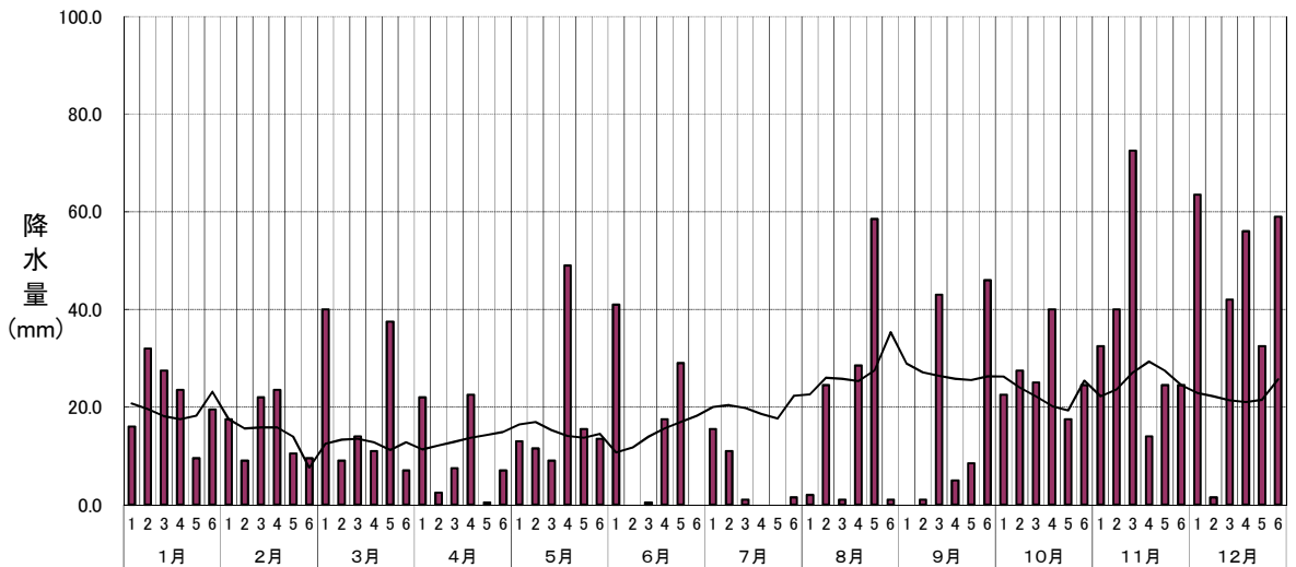
半旬別気象図 降水量(市浦:2021年)
