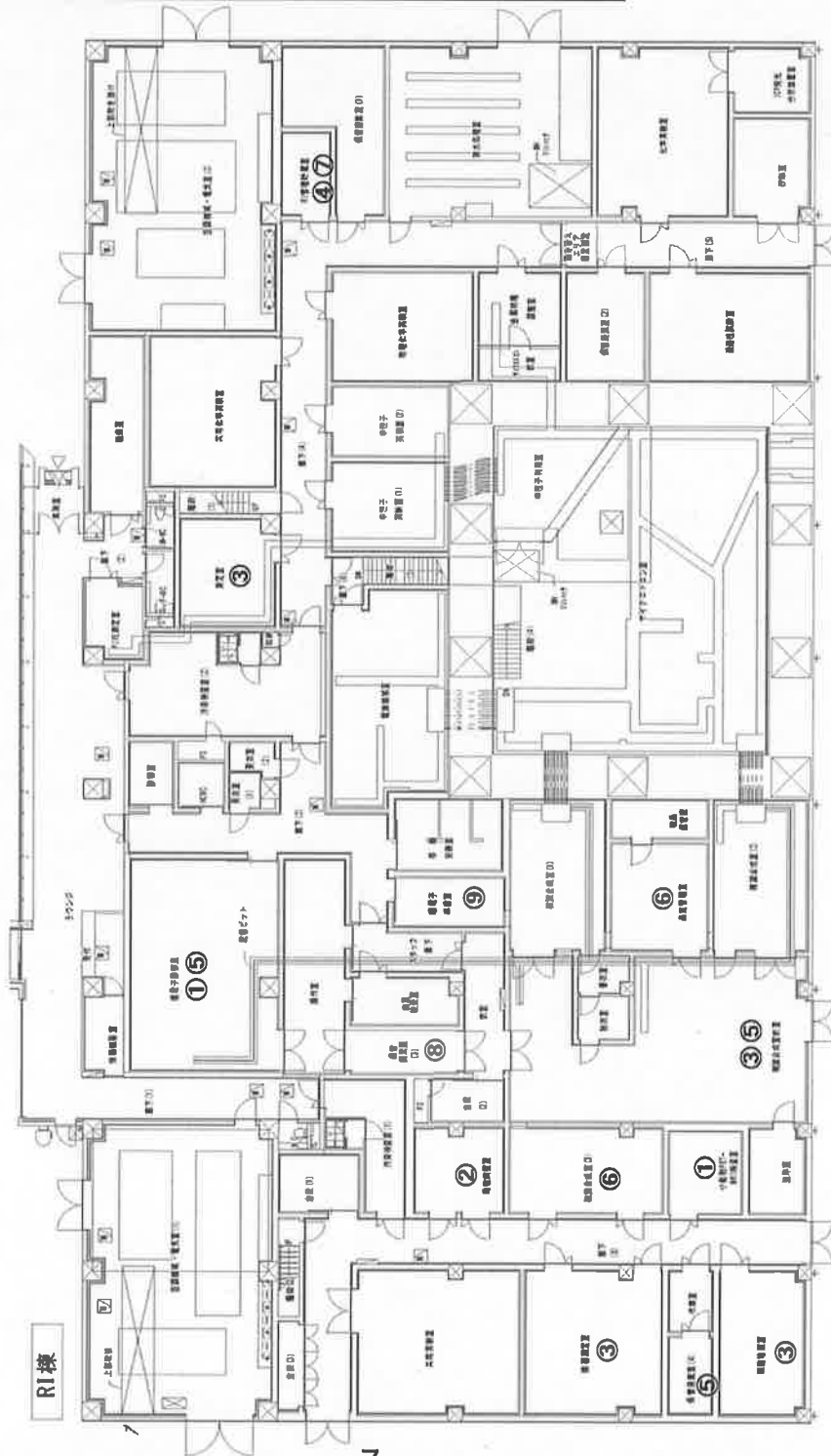
別図1 配置図
