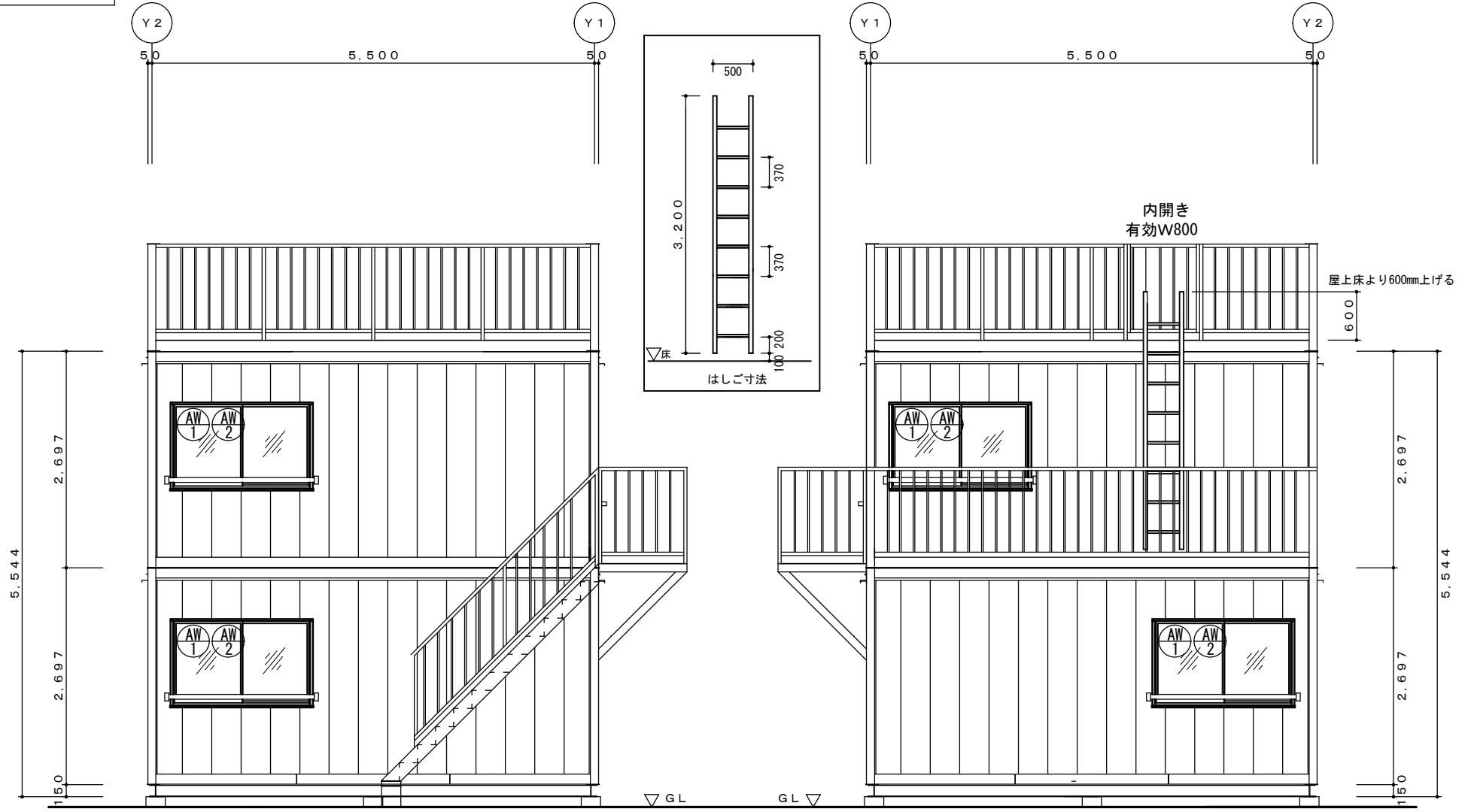
X 1-立面図 S=1/50
