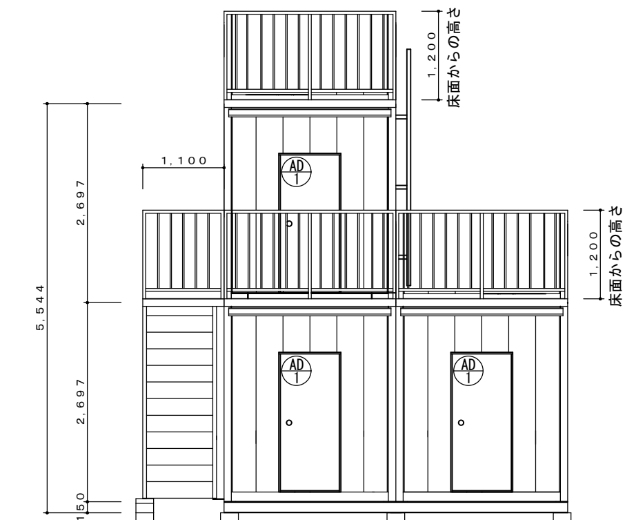
Y 1-立面図 S=1/50
