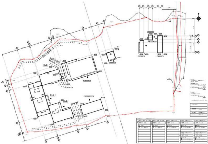
配置図
